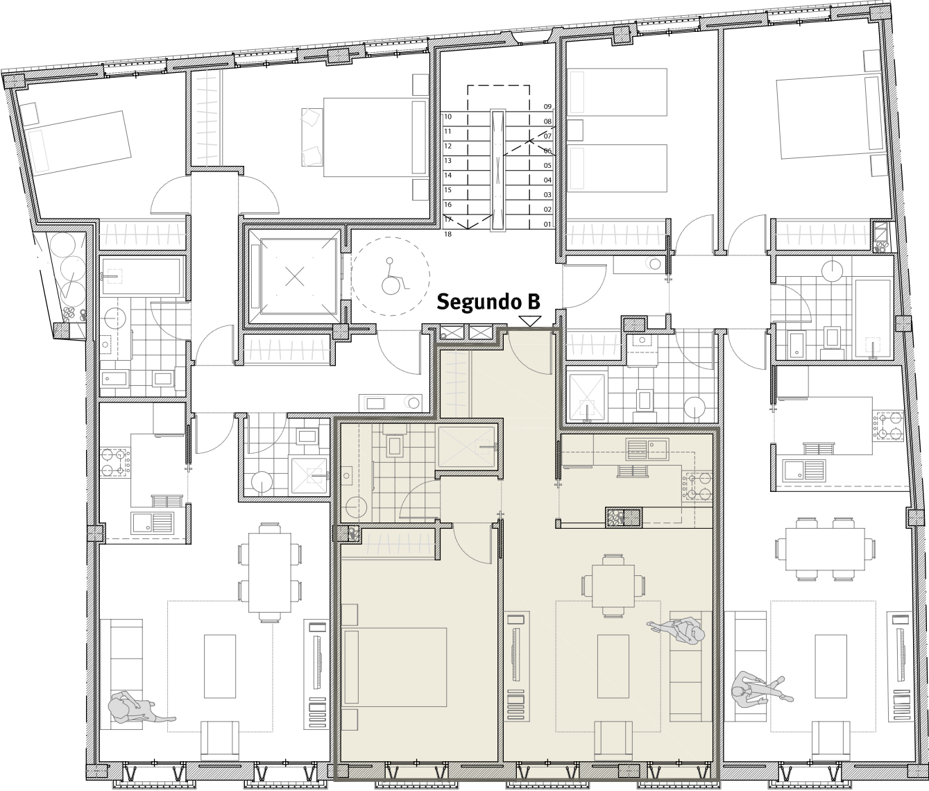
PLANTA SEGUNDA
