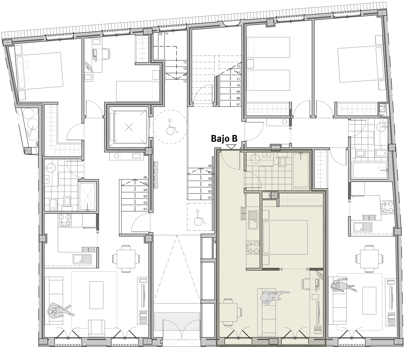
PLANTA BAJA
