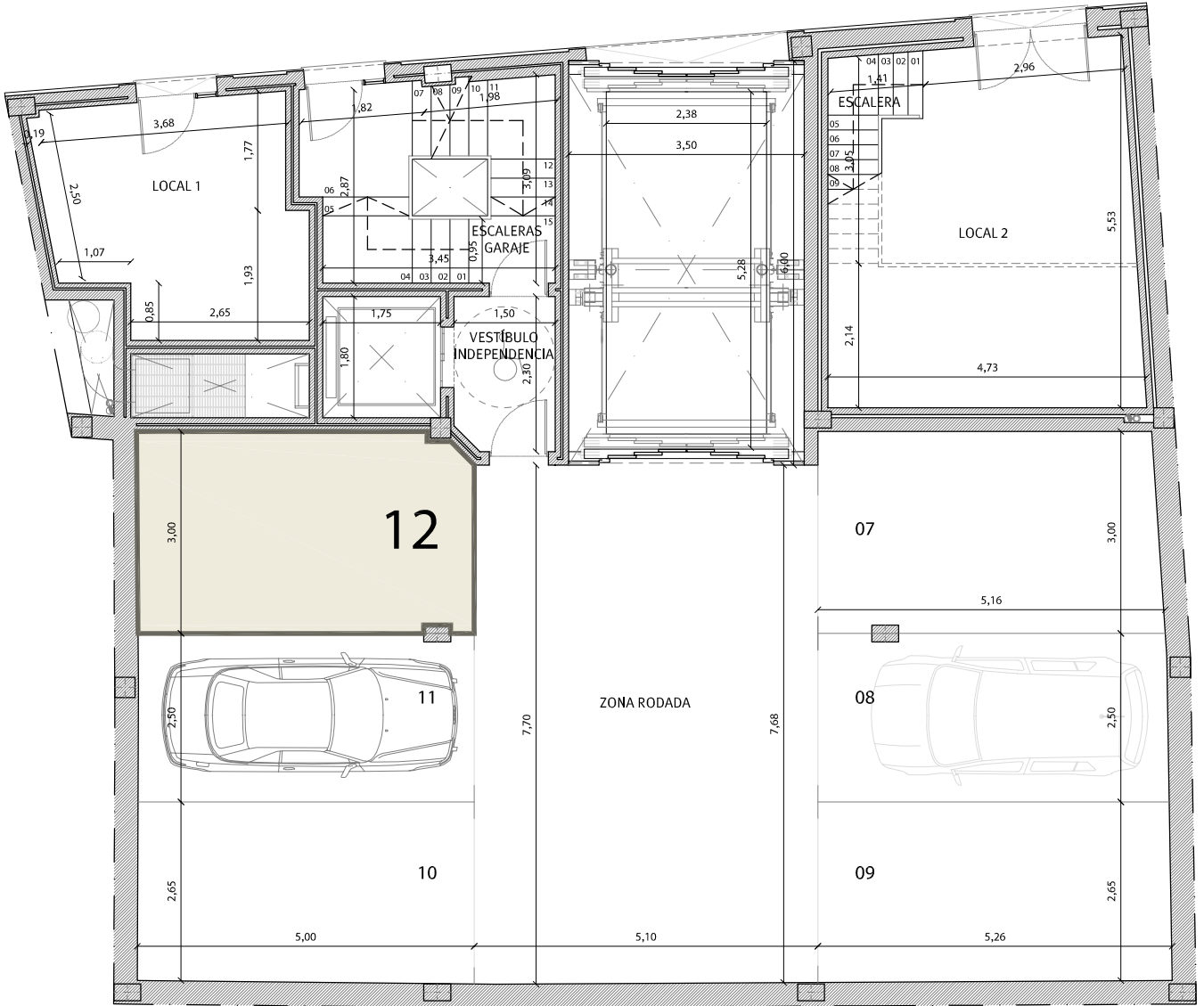
PLANTA SÓTANO 2
